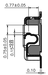
SECTION A-A (SCALE 2:1)
